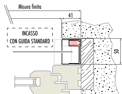
SEZ. B-B
