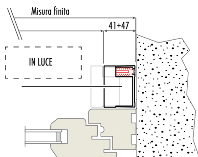
SEZ. B-B
