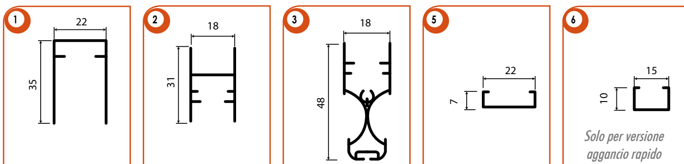
Laterale con chiusura a magneti
