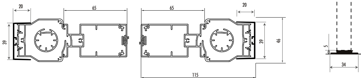
Centrale RollOut Magnum
