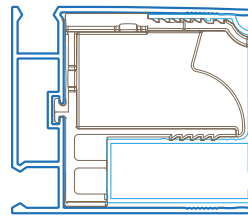
Kit Reggi guida 20 A con tecnologia TURN & FIX | OPTIONAL
