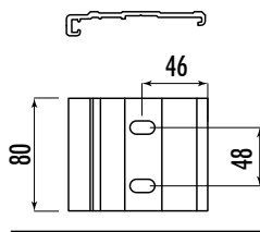
Supporto a soffitto Ceiling support
