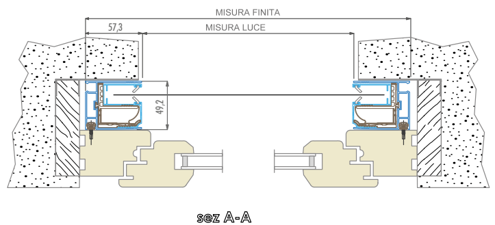
Kit Reggi guida 22 A con tecnologia TURN & FIX | OPTIONAL
