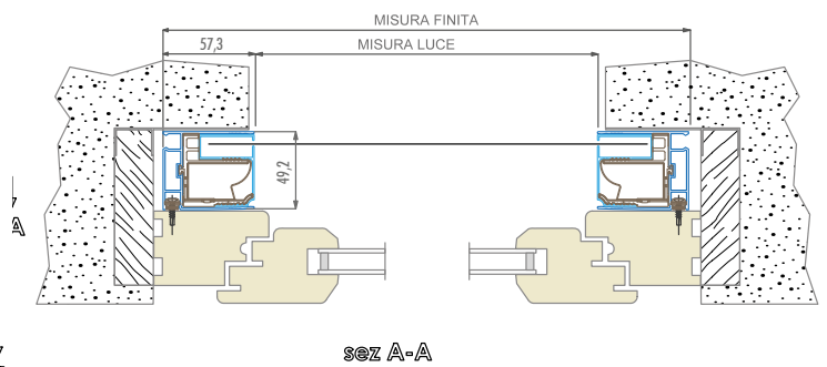
Kit Reggi guida 20 A con tecnologia TURN & FIX | OPTIONAL
