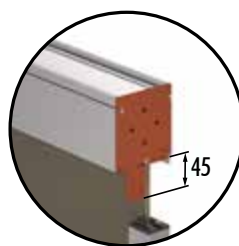
TV Testata con viti laterali Head with lateral screws
