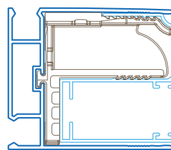
Kit Reggi guida 22 A con tecnologia TURN & FIX | OPTIONAL
