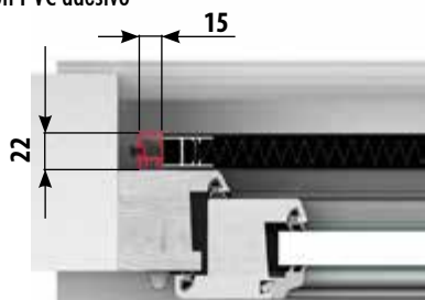
Fissaggio con PVC adesivo
