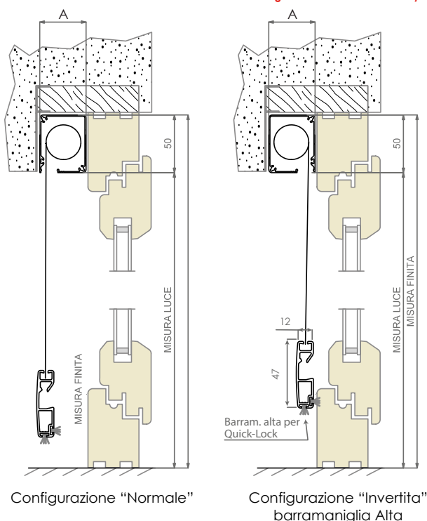
sez A-A
