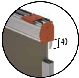
Testata con perno centratore Head with center pin
