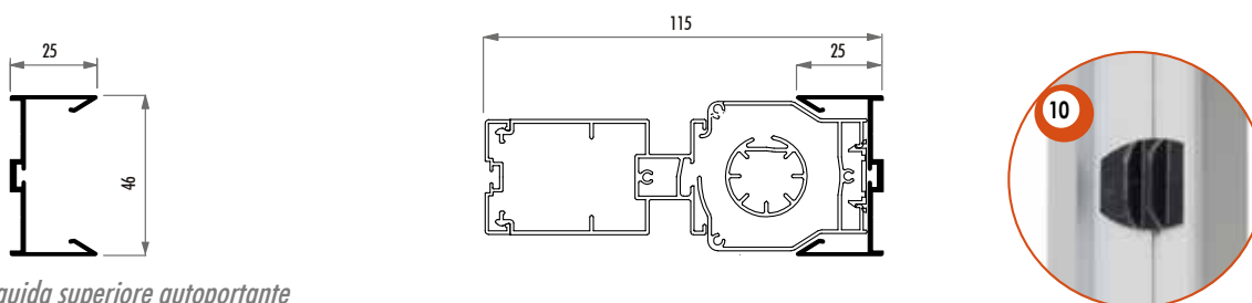
Centrale RollOut Magnum
