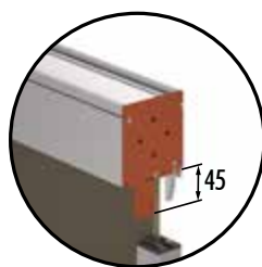
TCV Testata con perno centratore e viti laterali Head with pin and lateral screws
