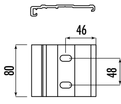
Supporto a soffitto Ceiling support
