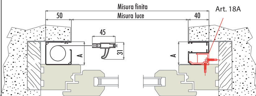
SEZ. B-B
